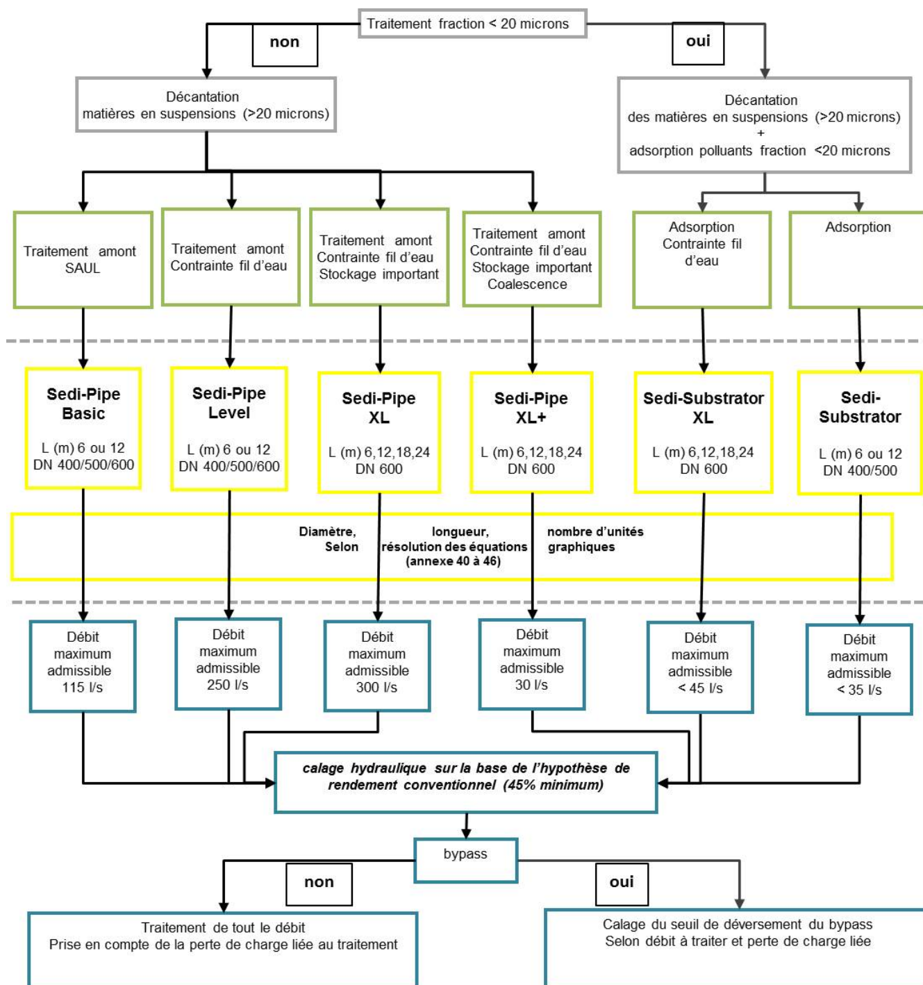
Figure 32 : Logigramme de choix et dimensionnement Sedi-pipe
