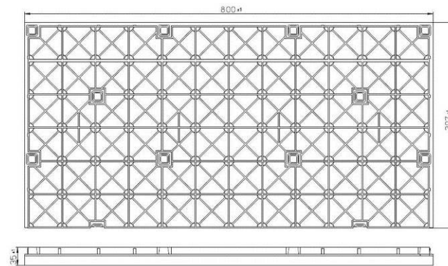
Figure 7 : grille anti remobilisation / coalescence
