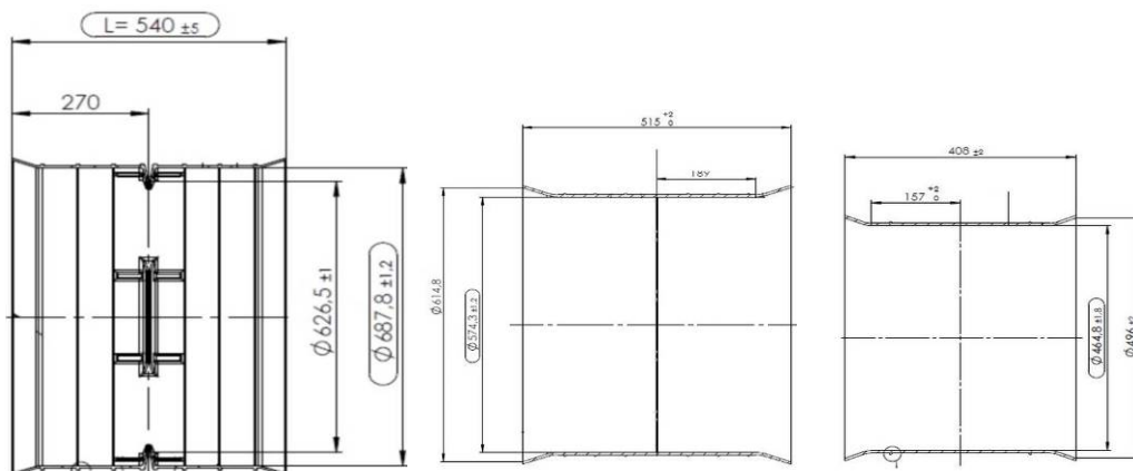
Figure 7 : grille anti remobilisation / coalescence
