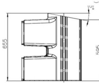
Figure 18 : Détail pièce de jonction SAUL Rigofill
