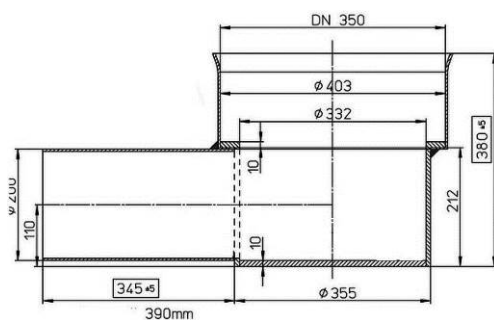
Figure 24 : Détail pièce de jonction cartouche Sedi-substrator
