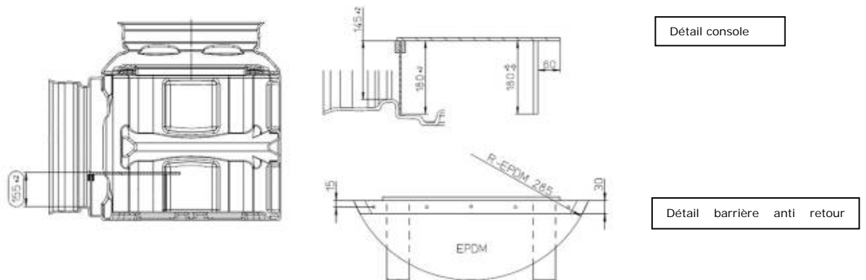
Figure 13 : Élément de fond de la boîte d'inspection départ Sedi-pipe basic /level pour tube de sédimentation entrée DN 500
